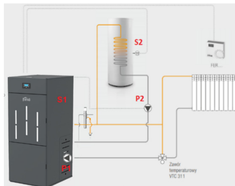
Rys.1 Podłączenie z dwiema pompami
