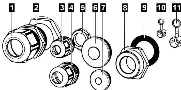
Rys. 3-2: Materiał montażowy
