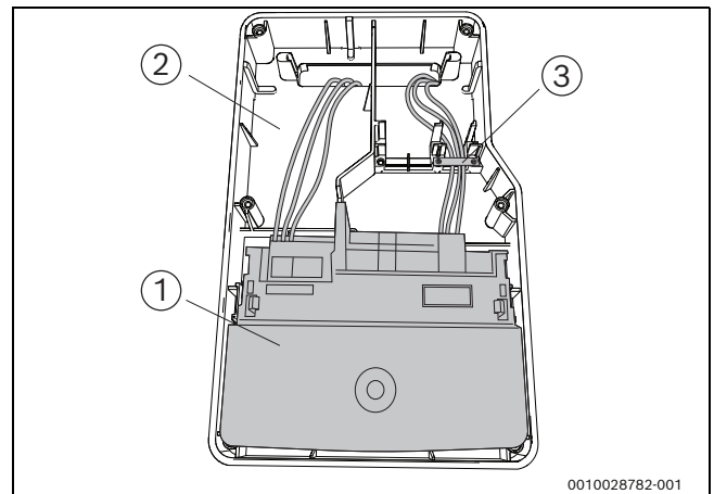
Rys. 52 Zainstalować moduł funkcyjny w skrzynce modułu
