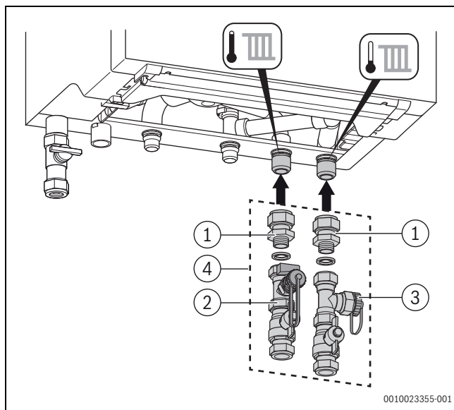
Rys. 24 Podłączenie rur wody grzewczej do urządzenia
