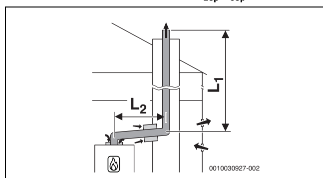
Rys. 44 Sztywne odprowadzenie spalin w szachcie wg B 23p /B 53p z zależnym od powietrza w pomieszczeniu doprowadzeniem powietrza do urządzenia i koncentryczną złączką między pomieszczeniem zainstalowania a szachtem
