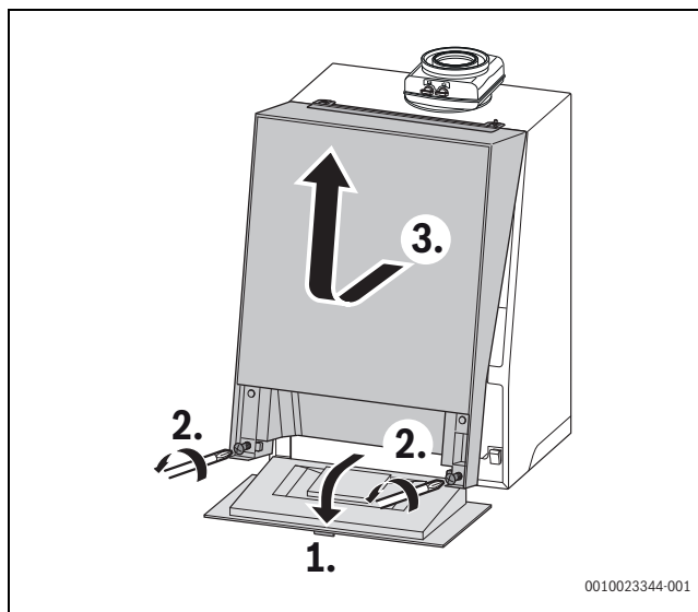
Rys. 19 Demontaż obudowy urządzenia
