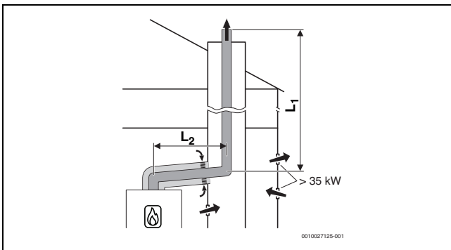
Rys. 46 Sztynne odprowadzenie spalin w szachcie wg B 33 z zależnym od powietrza w pomieszczeniu doprowadzeniem powietrza przez koncentryczną instalację powietrzno-spalinową w pomieszczeniu zainstalowania
