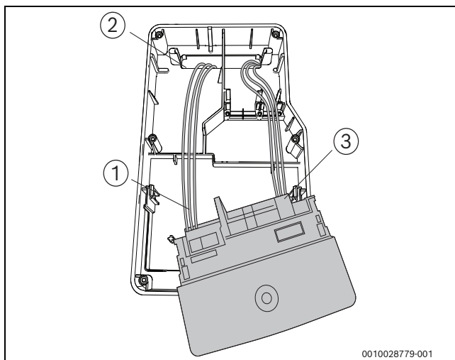
Rys. 51 Funktionsmodul anschließen
