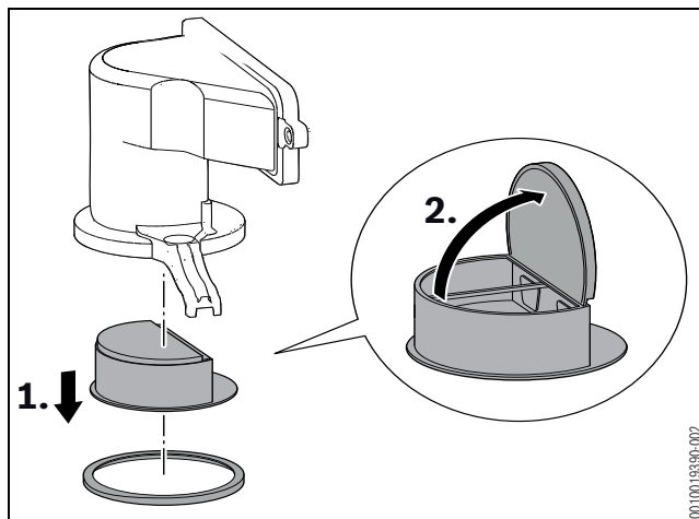
Rys. 74 Zawór klapowy zwrotny w urządzeniu mieszającym
