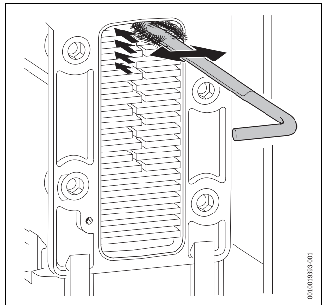
Rys. 77 Czyszczenie bloku cieplnego szczotką
