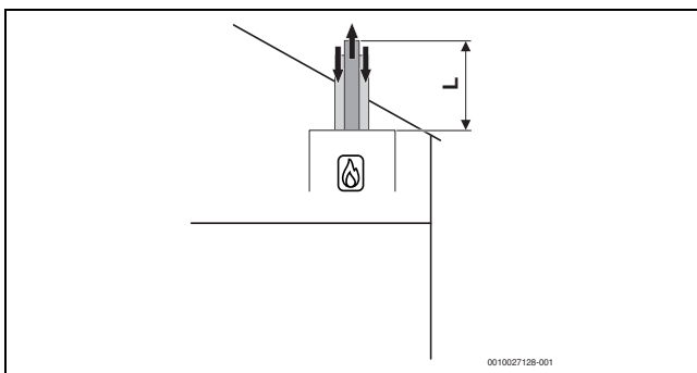
Rys. 38 Pionowa koncentryczna instalacja powietrzno-spalinowa wg C 33x
