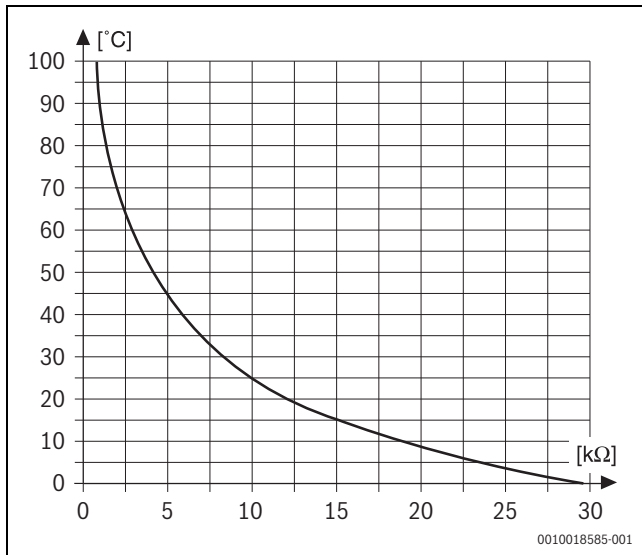
Rys. 10 Charakterystyka rezystancji czujników temperatury (nie dotyczy czujników temperatury zewnętrznej)
