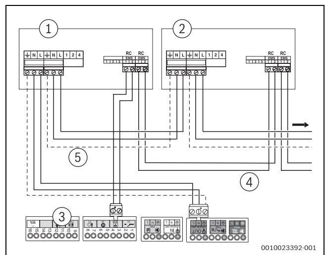
Rys. 53 Podłączenie kilku modułów funkcyjnych
