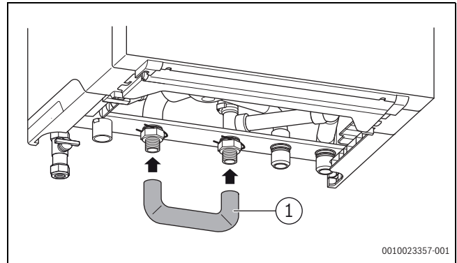
Rys. 28 Eksploatacja bez podgrzewacza pojemnościowego c.w.u.
