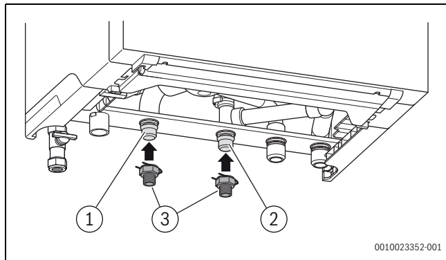
Rys. 21 Montaż przewodów rurowych dla podgrzewacza pojemnościowego c.w.u. T40S
