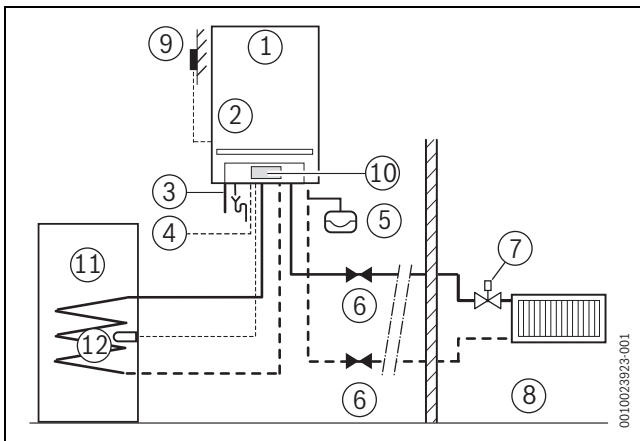
Rys. 27 Przykład instalacji z regulacją wg temperatury zewnętrznej i podgrzewaczem pojemnościowym c.w.u.
