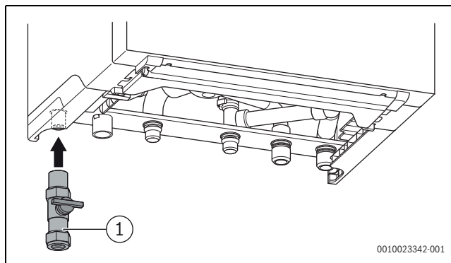
Rys. 18 Wykonanie przyłącza gazowego
