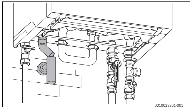
Rys. 31 G-TA Syfon kondensatu (osprzęt)
