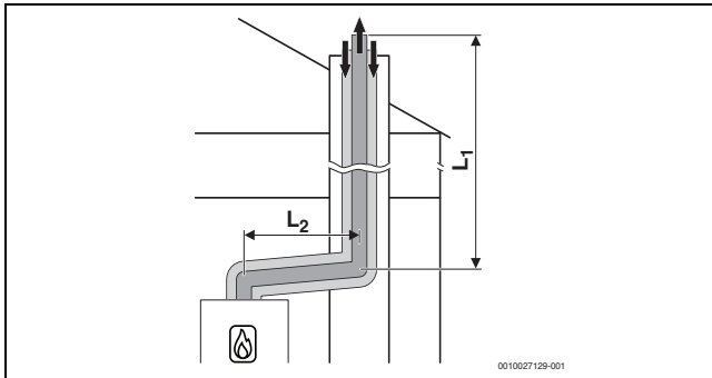
Rys. 37 Koncentryczna instalacja powietrzno-spalinowa wg C 33x w szachcie
