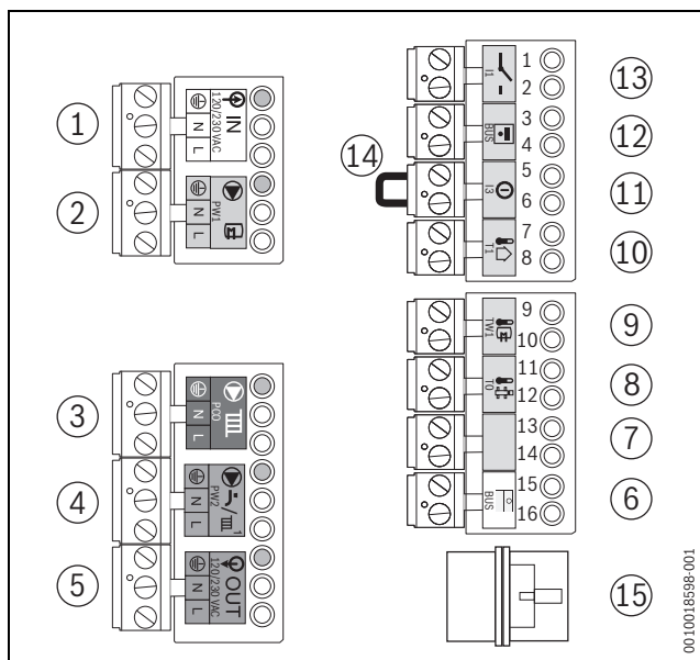
Rys. 50 Listwy zaciskowe
