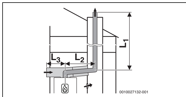
Rys. 40 Szytowe odprowadzenie spalin C 53x w szachcie i instalacja powietrzno-spalinowa z oddzielnym doprowadzeniem powietrza i koncentrycznym odprowadzeniem spalin w pomieszczeniu zainstalowania
