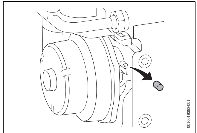
Rys. 76 Króciec pomiarowy na urządzeniu mieszającym
