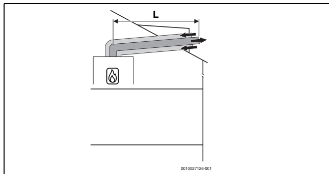
Rys. 35 Pozioma koncentryczna instalacja powietrzno-spalinowa C 13x przez dach
