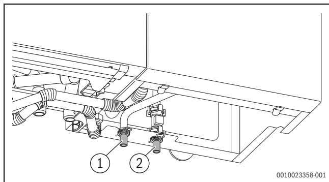
Rys. 30 Przyłącza wody
