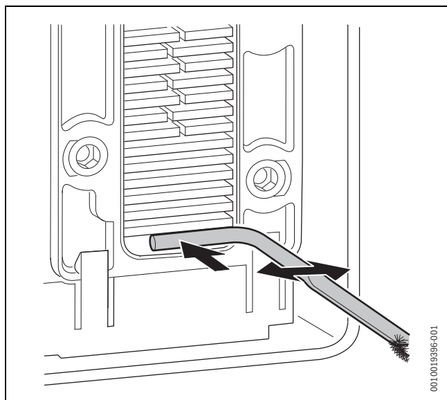
Rys. 79 Czyszczenie wanny kondensatu
