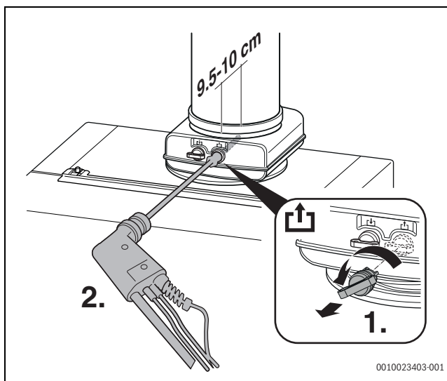
Rys. 58 Pomiar zawartości CO/CO 2
