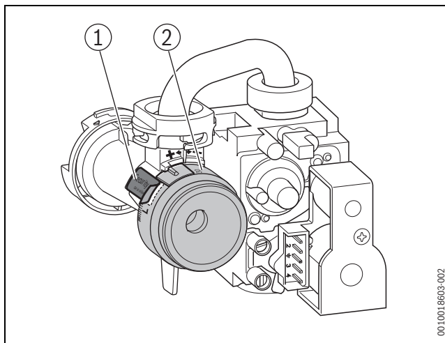
Rys. 57 Usuwanie naklejki
