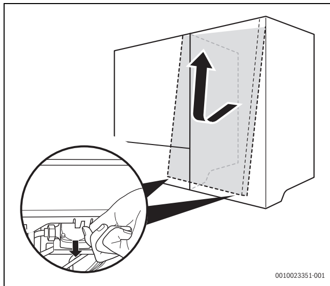
Rys. 20 Demontaż obudowy zasobnika warstwowego c.w.u.
