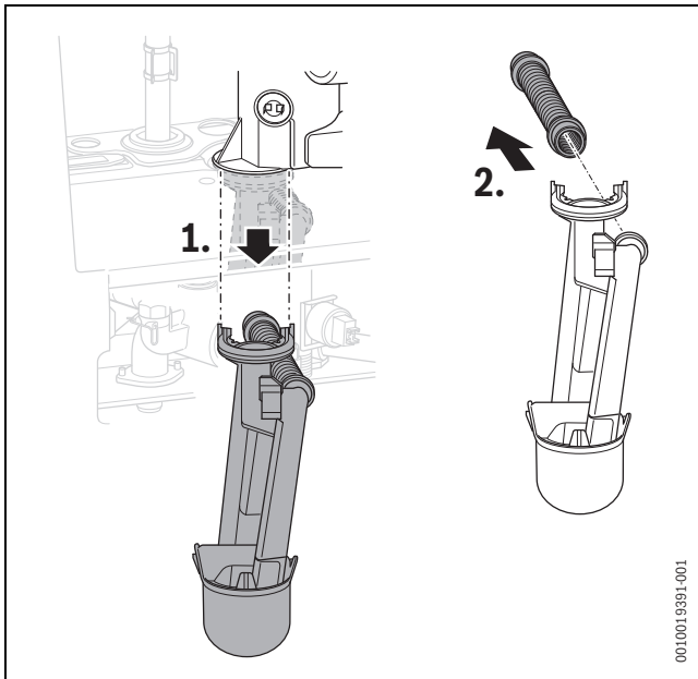
Rys. 75 Syfon kondensatu
