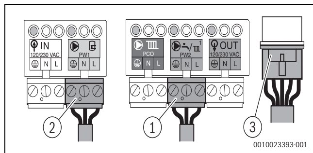
Rys. 54 Podłączenie podgrzewacza pojemnościowego c.w.u. T40S
