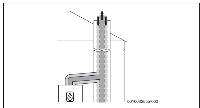
Rys. 39 Koncentryczna instalacja powietrzno-spalinowa wg C 43x w pomieszczeniu zainstalowania
