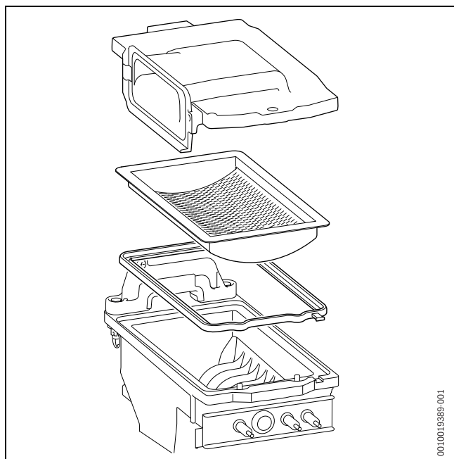
Rys. 72 Wymywanie palnika
