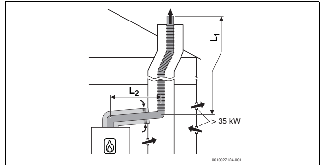
Rys. 47 Elastyczne odprowadzenie spalin w szachcie wg B 33 z zależnym od powietrza w pomieszczeniu doprowadzeniem powietrza przez koncentryczną instalację powietrzno-spalinową w pomieszczeniu zainstalowania
