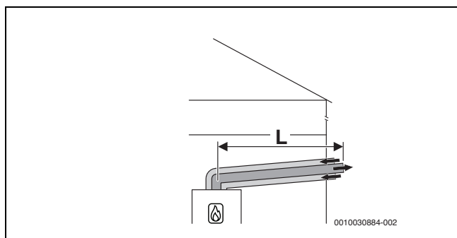
Rys. 36 Pozioma koncentryczna instalacja powietrzno-spalinowa C 13x przez ścianę zewnętrzną
