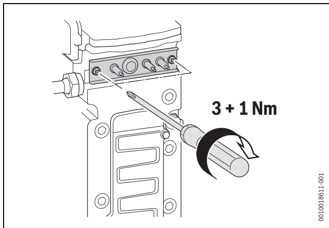
Rys. 69 Montaż zestawu elektrod
