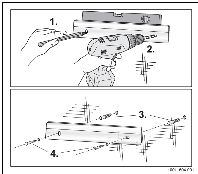
Rys. 15 Montaż uchwyty naściennego
