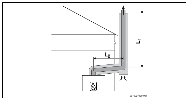
Rys. 41 Koncentryczna instalacja powietrzno-spalinowa wg C 53x na ścianie zewnętrznej
