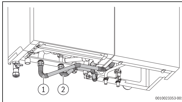
Rys. 22 Połączenie podgrzewacza pojemnościowego c.w.u. T40S z urządzeniem
