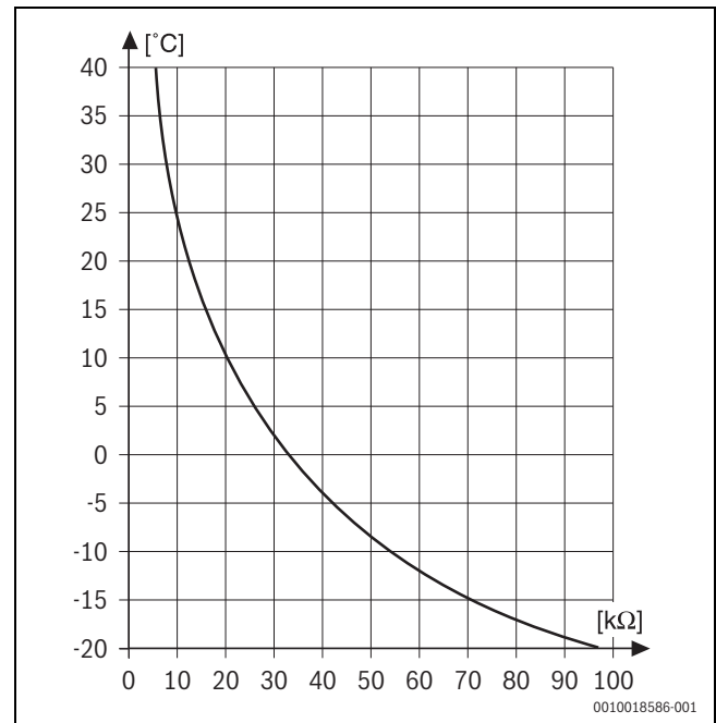
Rys. 11 Charakterystyka rezystancji dla czujników temperatury zewnętrznej
