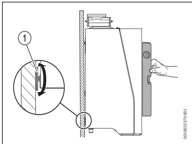
Rys. 16 Wyrównywanie urządzenie
