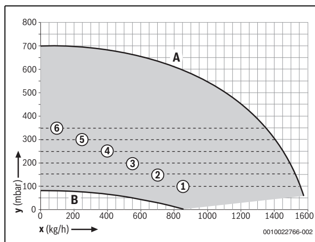
Rys. 8 15-35 kW: Ciśnienie dyspozycyjne dla ustawienia 1 - 6
