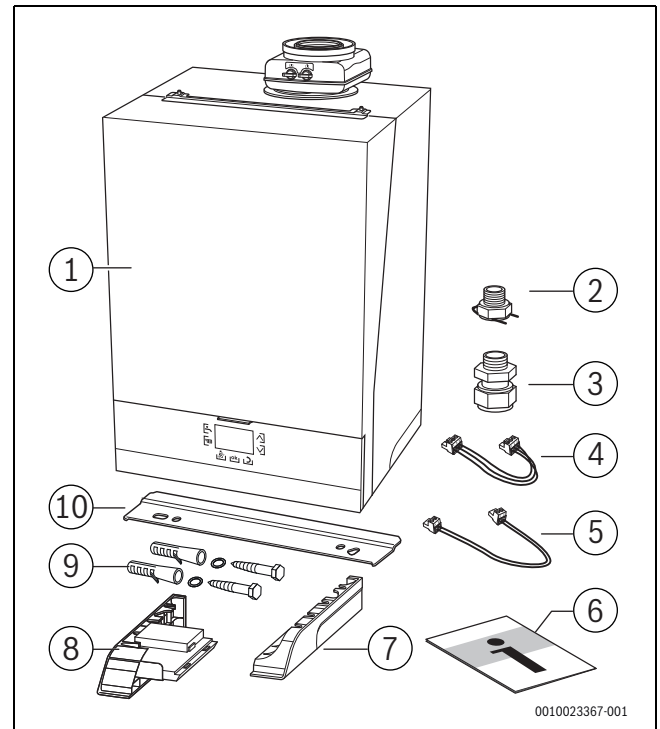
Rys. 1 Zakres dostawy
