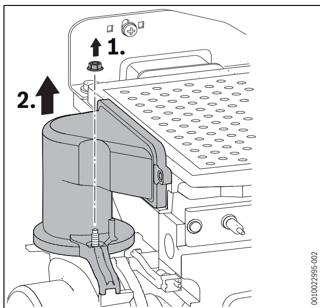
Rys. 73 Wymywanie urządzenie mieszające
