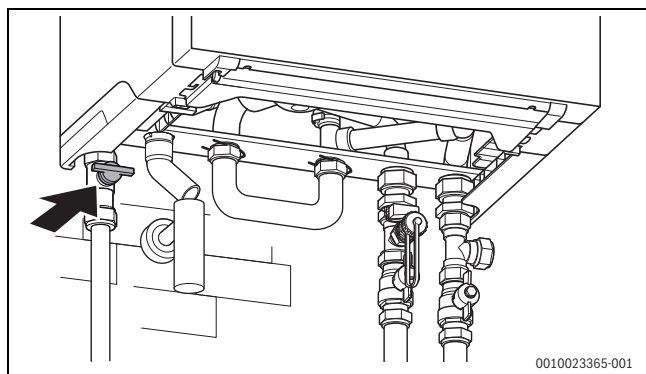
Rys. 66 Zamknięcie kurka gazowego
