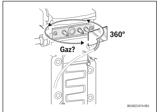
Rys. 70 Próby szczelności
