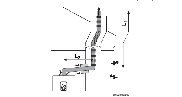
Rys. 45 Elastyczne odprowadzenie spalin w szachcie wg B 23p /B 53p z zależnym od powietrza w pomieszczeniu doprowadzeniem powietrza do urządzenia i koncentryczną złączką między pomieszczeniem zainstalowania a szachtem
