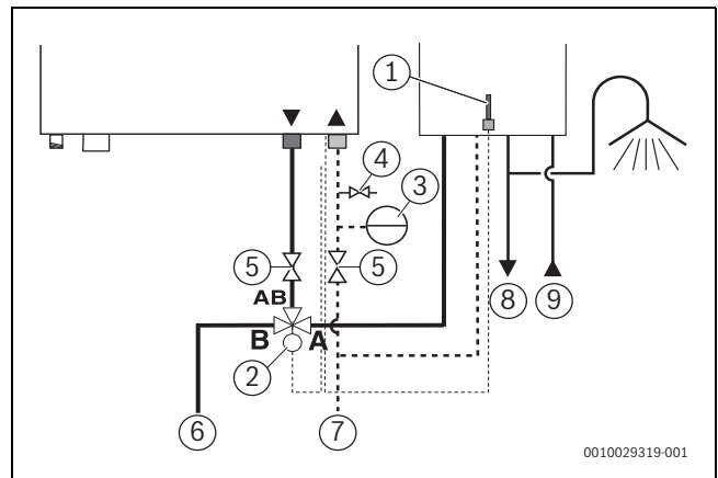
Rys. 29 Montaż zewnętrznego zaworu 3-drogowego (230 V)
